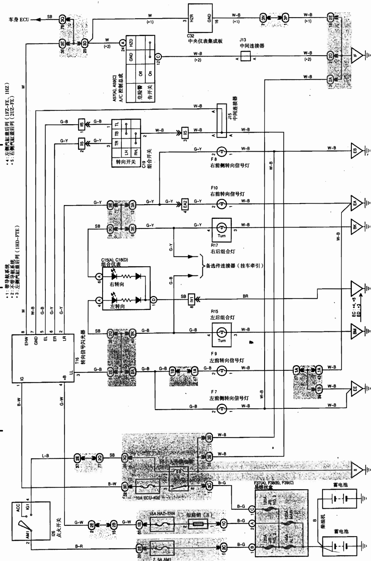
图 13-3-35 转向信号和应急警告灯电路图
